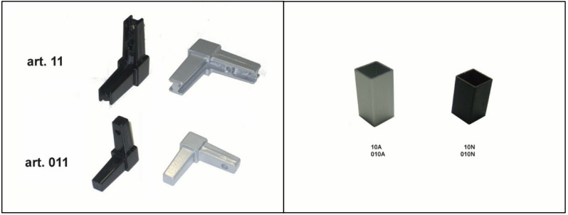
Sistema a tubolare 25x25 con giunti in metallo per la costruzine dei telai metallici
